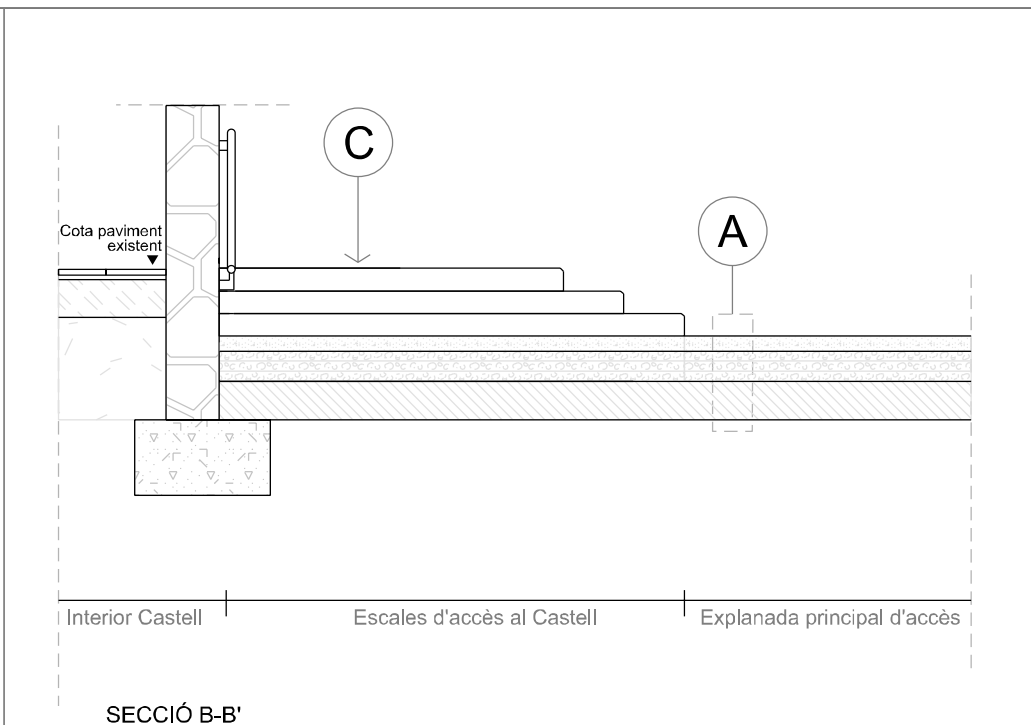
SECCIÓ B-B'
