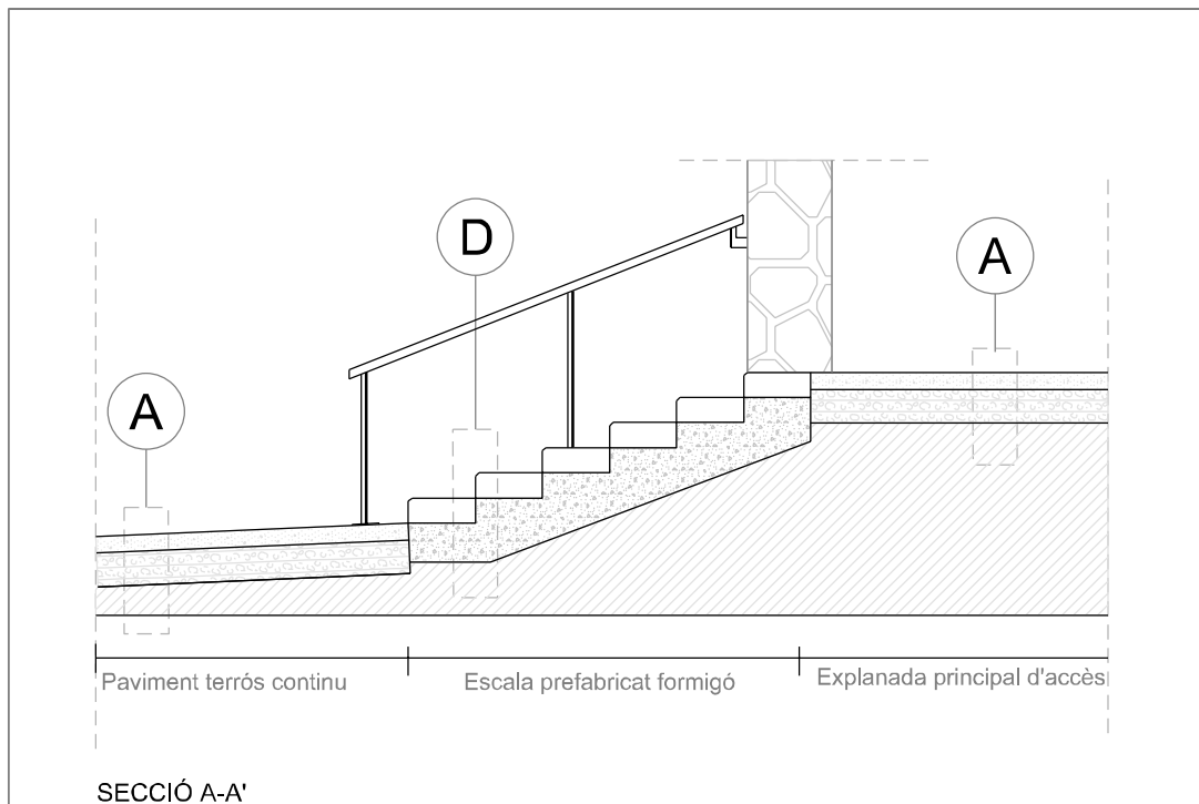
SECCIÓ A-A'
